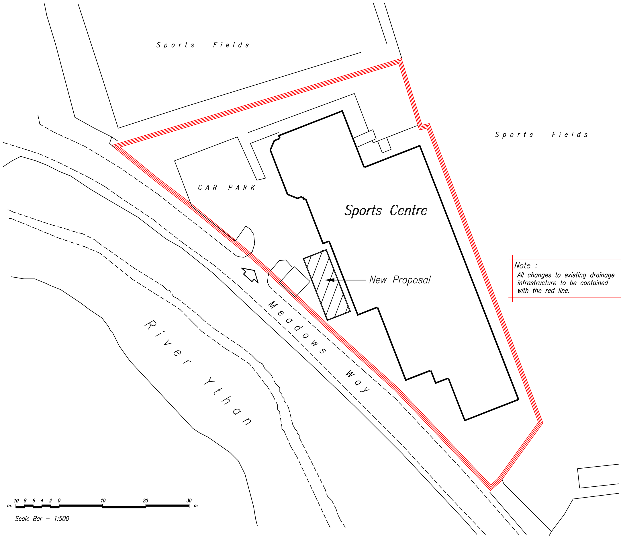
SITE LAYOUT PLAN : Scale 1:500
