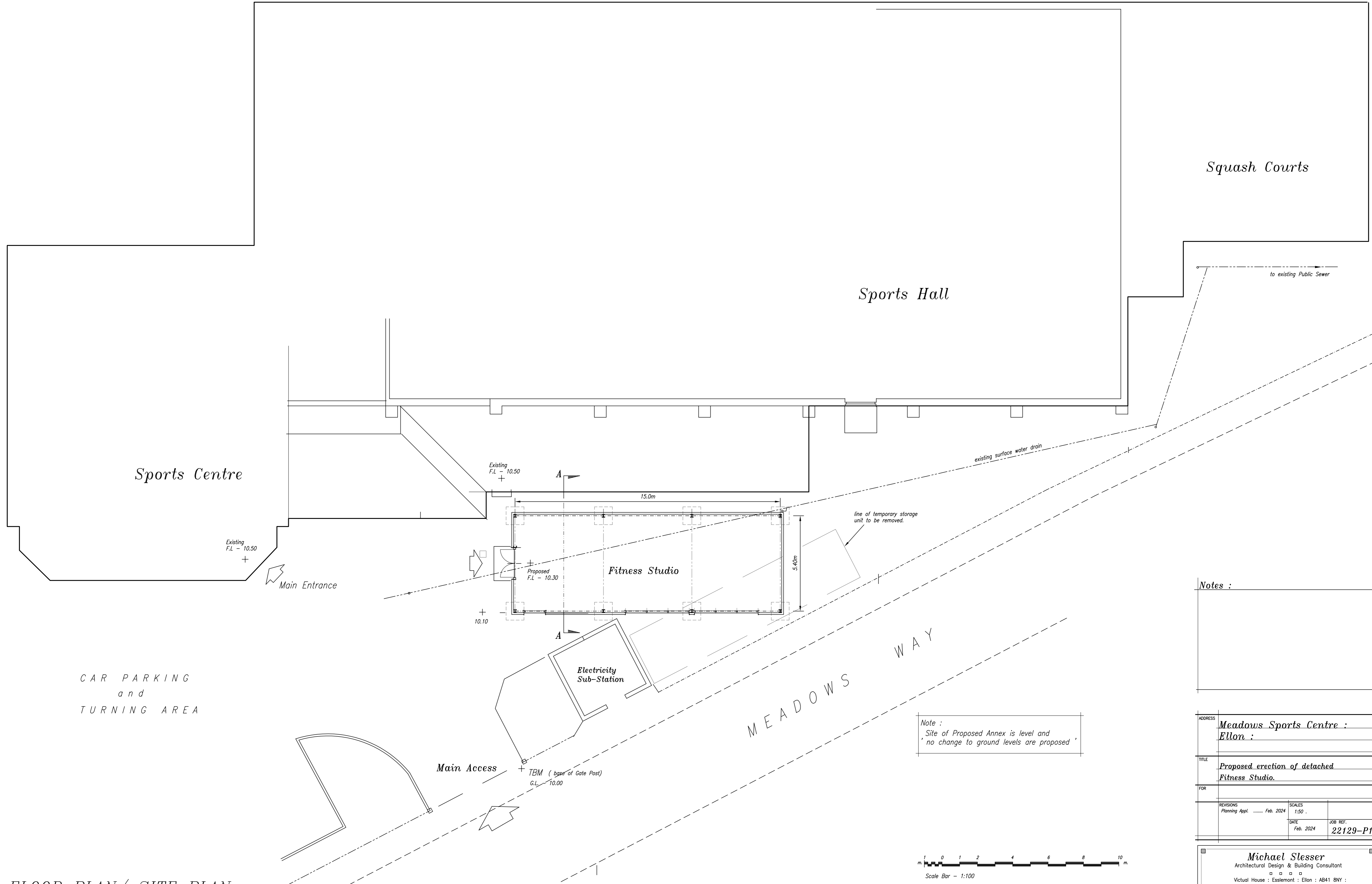
FLOOR PLAN/ SITE PLAN : Scale 1:100
