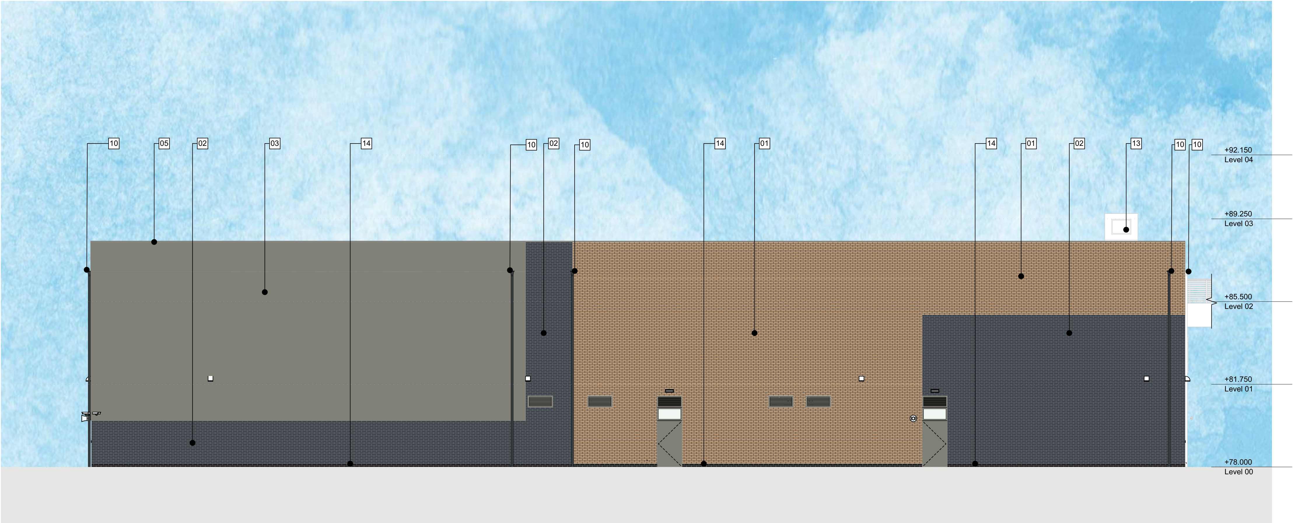
E-08 Elevation 'Hall West' 1:100
