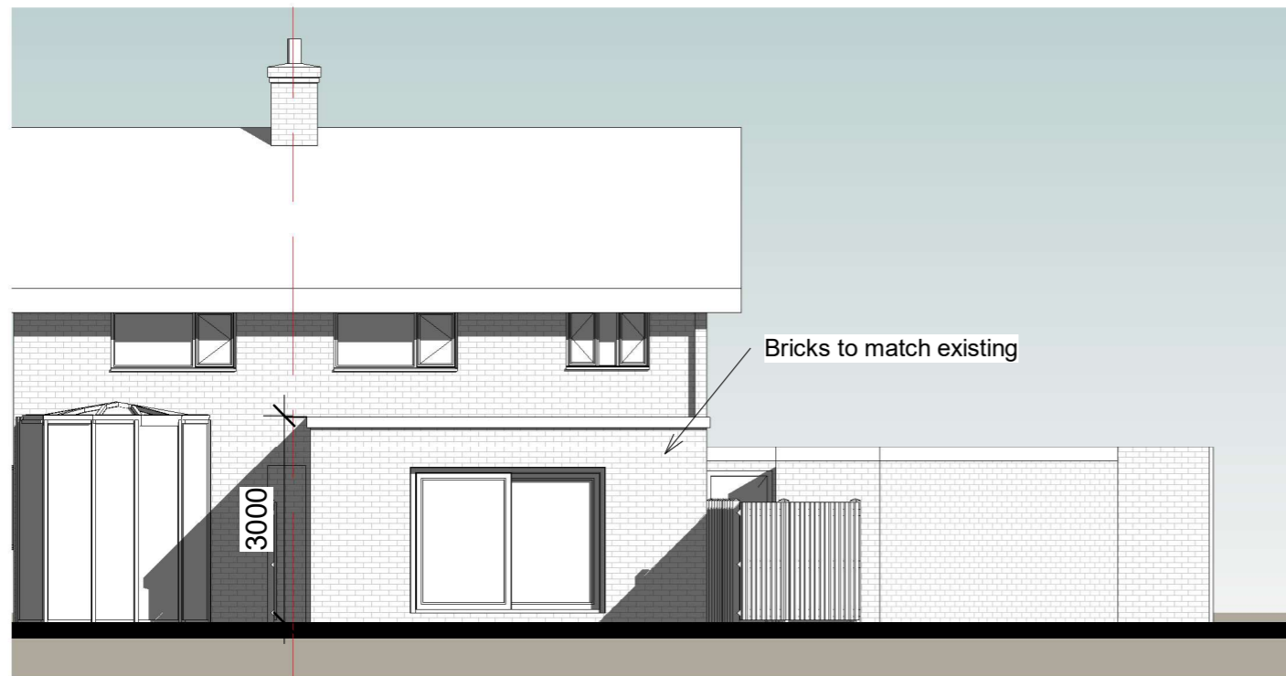
1 Back Elevation 1 : 100
