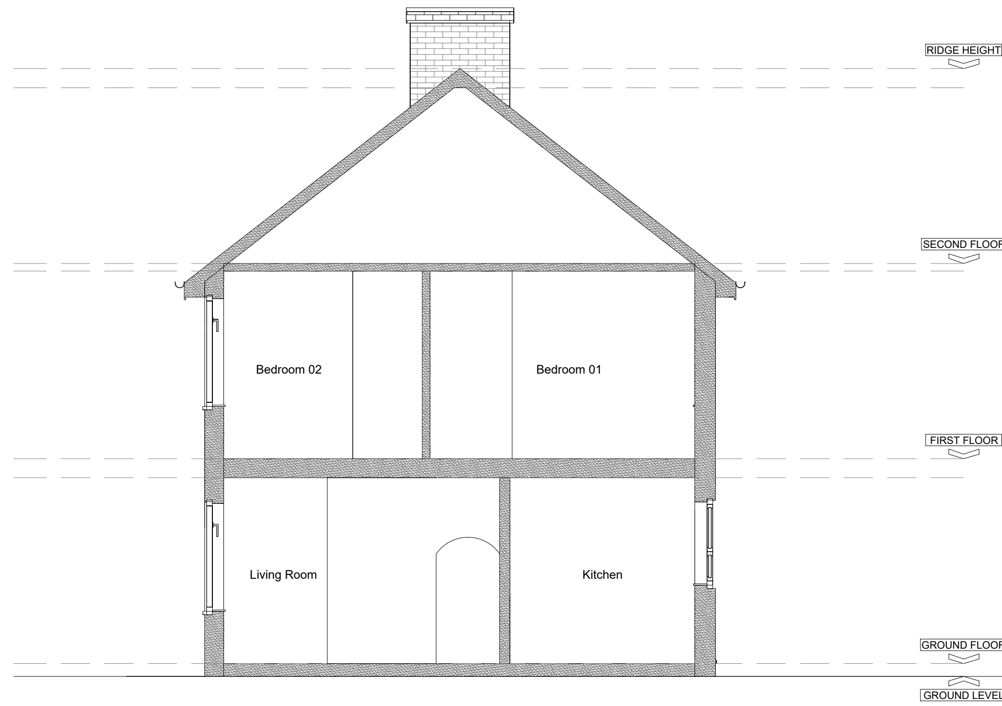
5 SECTION : A-A EXISTING 1:50 @ A1
