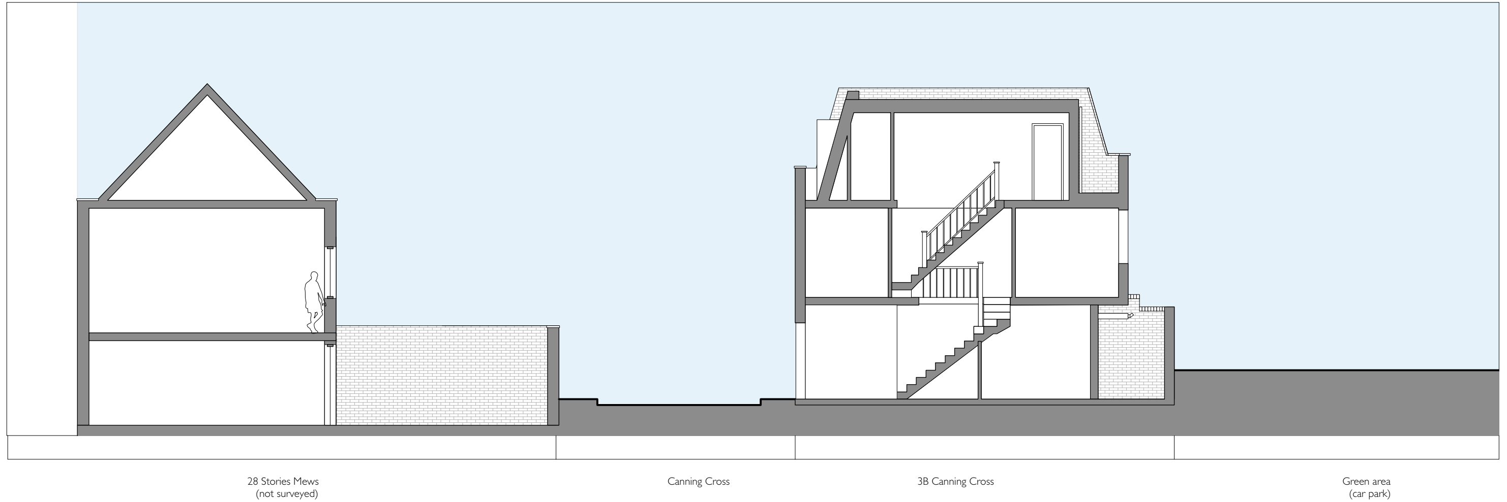
Existing Section AA Scale: 1:100
