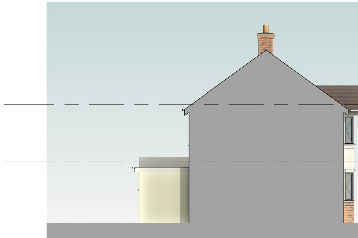
4 West 1 : 100
