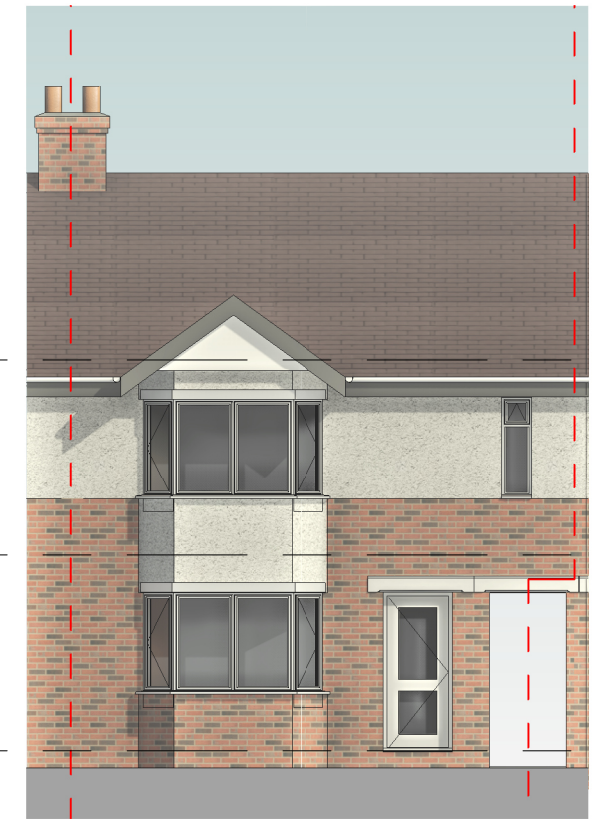
3 South 1 : 100
