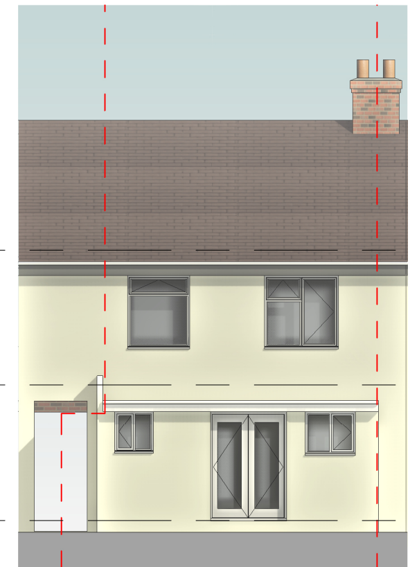
2 North 1 : 100
