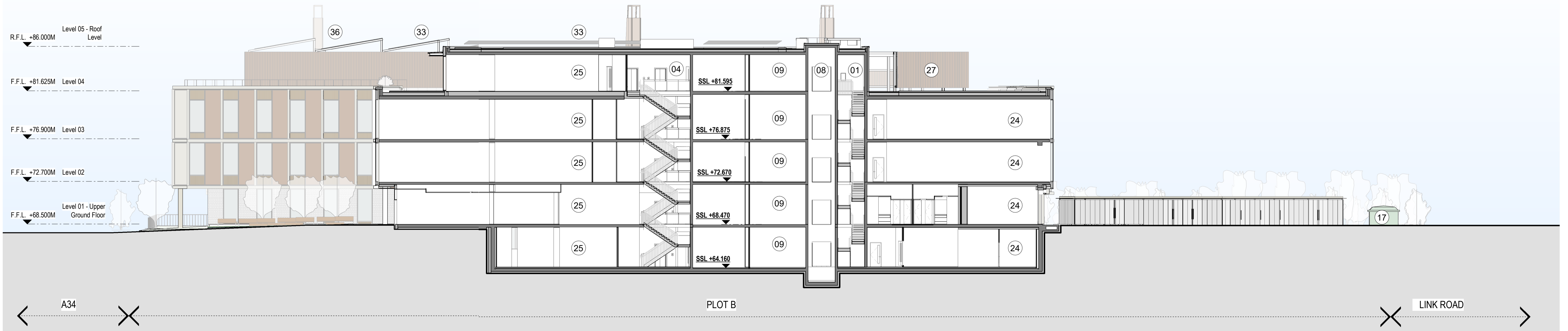
2 Section DD Central Core Long Section 1 : 200
