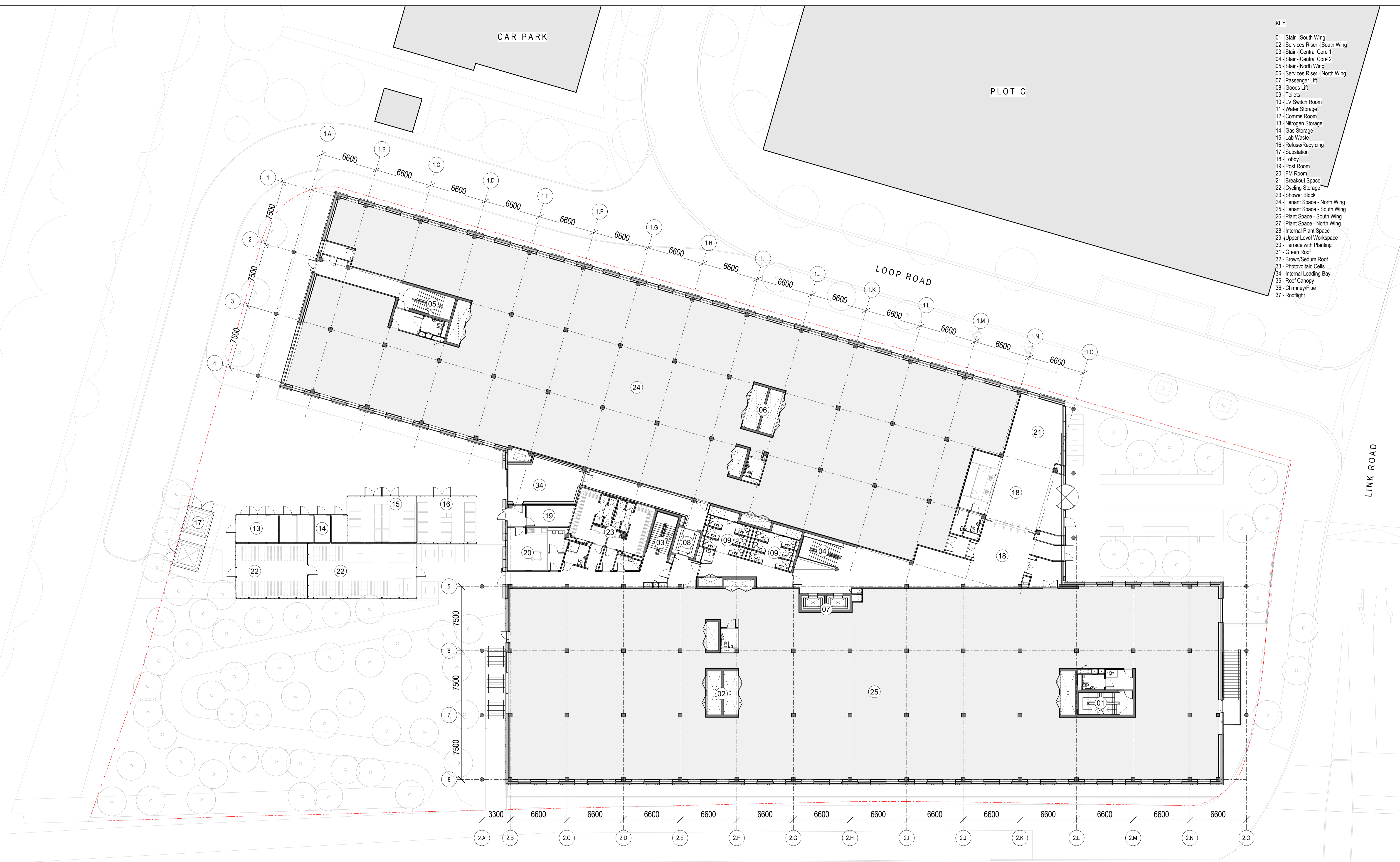
1 Level 01 - Plan 1 : 200
