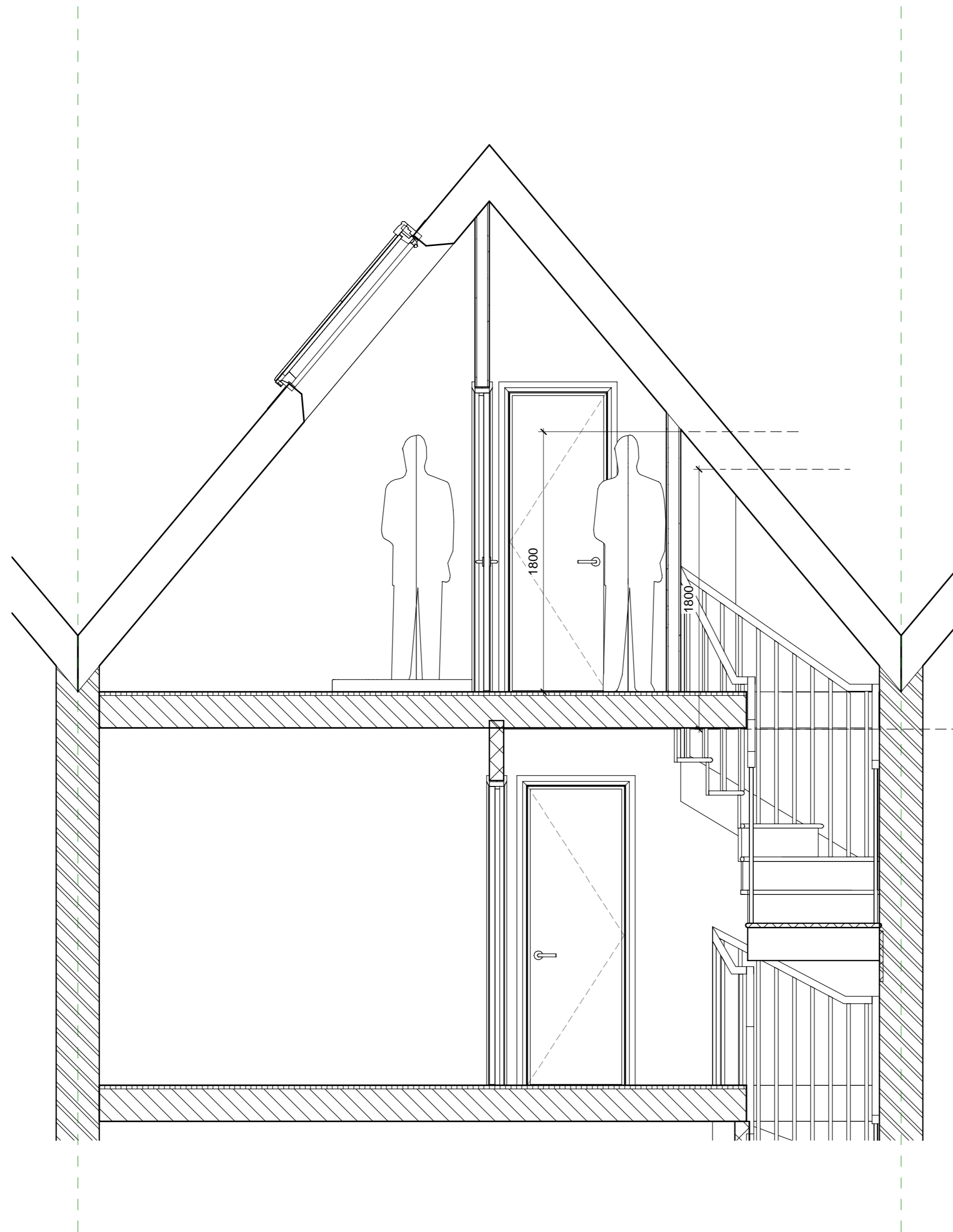
1 Loft Section 1 : 25
