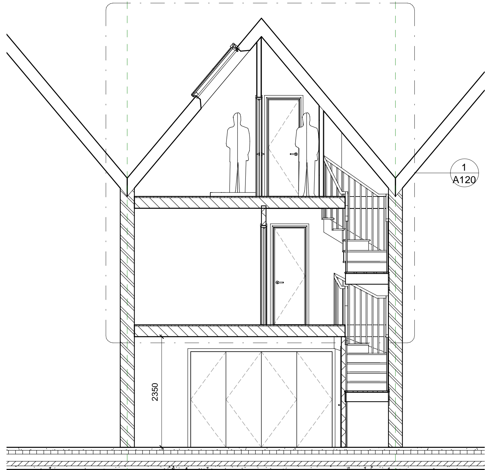
1 Section 2 1 : 50
