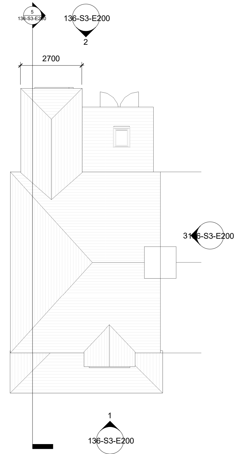
4 Roof Plan 1 : 100
