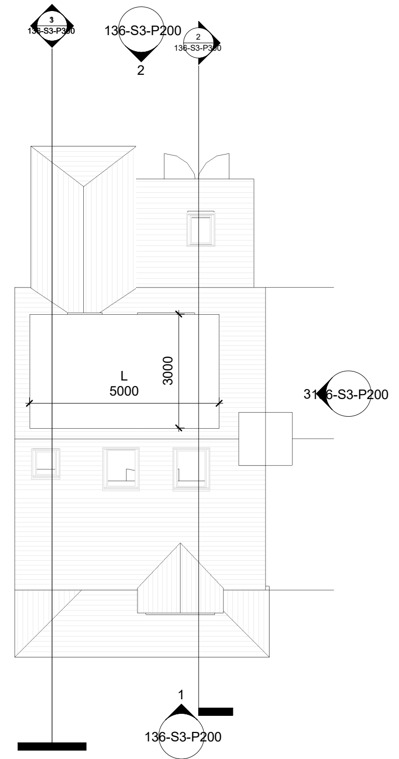
4 P- Roof Plan 1 : 100
