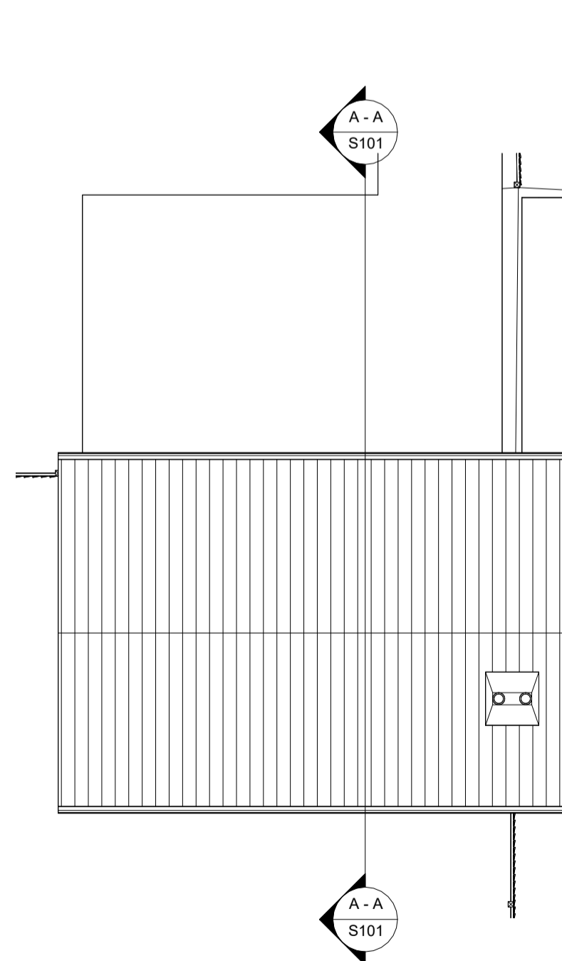
Roof Plan 1 : 100
