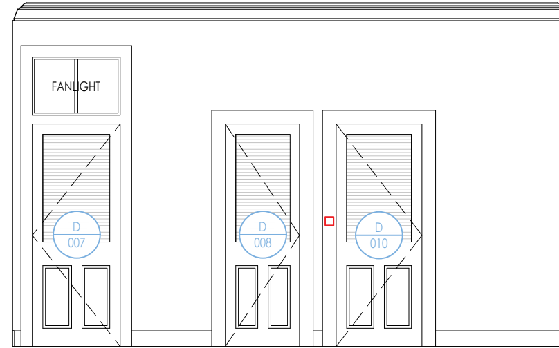
3_ELEVATION B 1:50 @ A3
