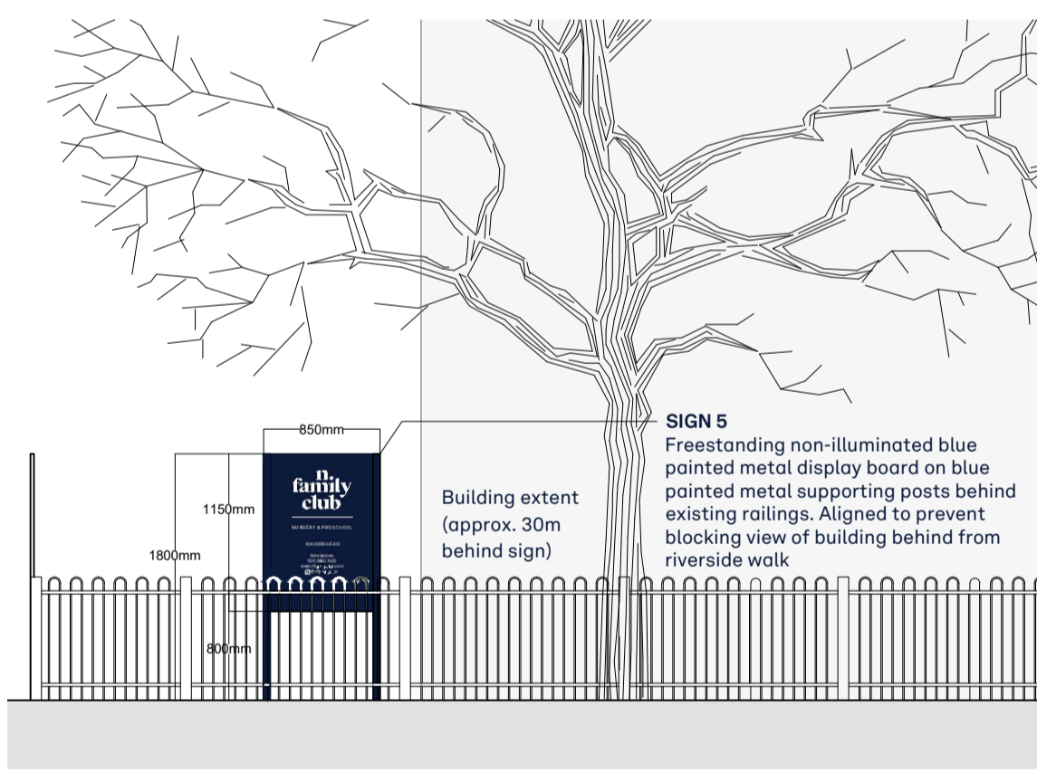
Elevation 5
