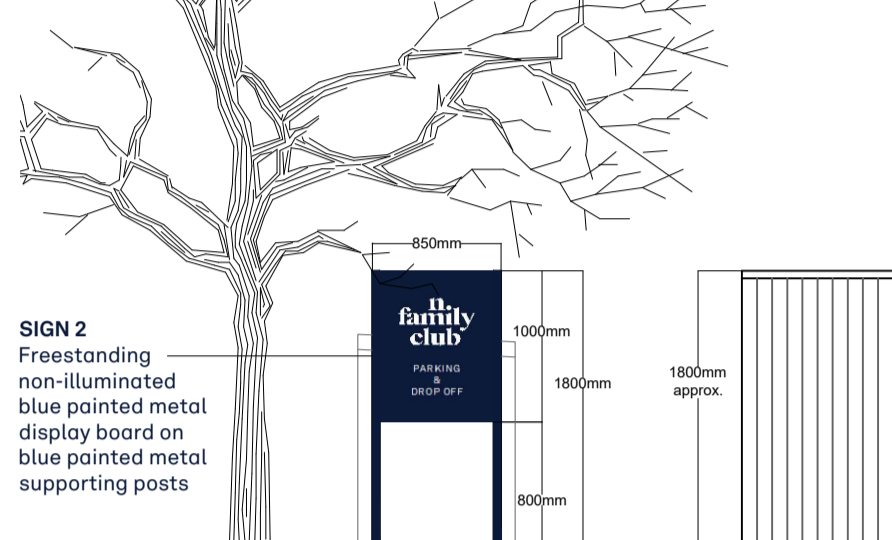
Elevation 2
