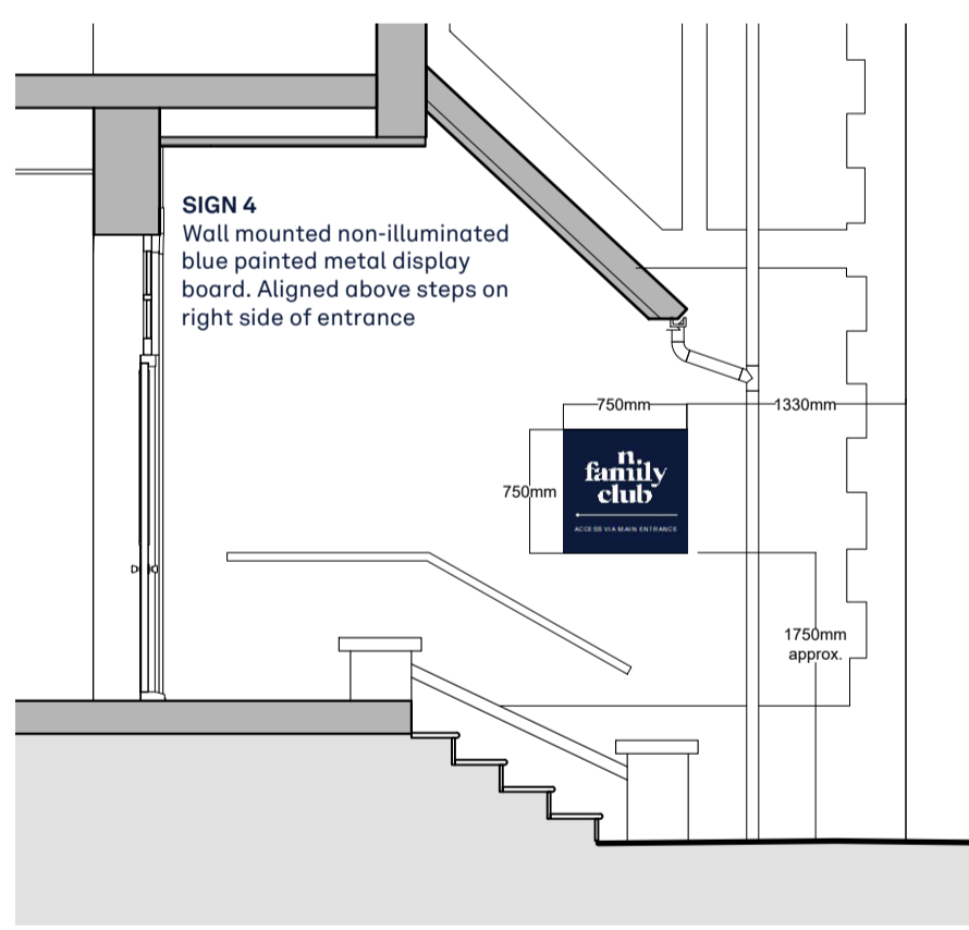
Elevation 4
