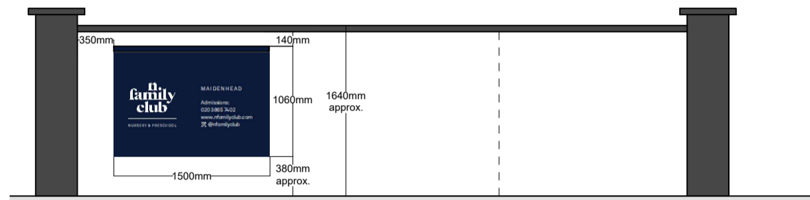
Elevation 1
