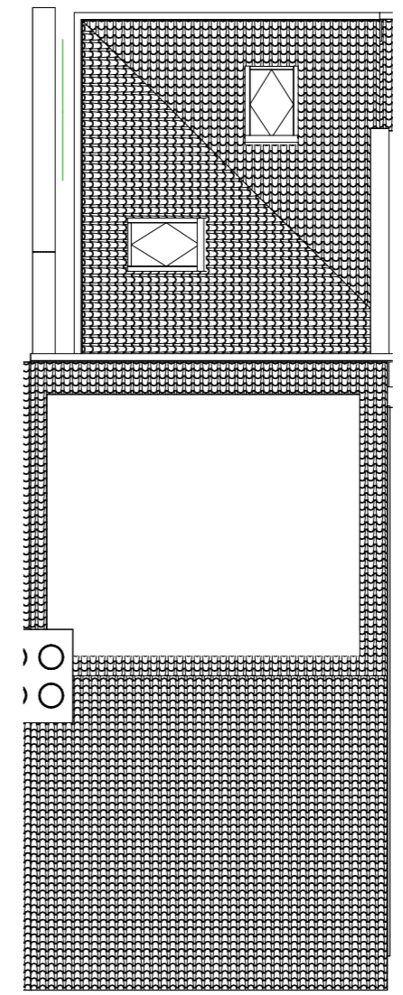
③ ROOF PLAN 1 : 100
