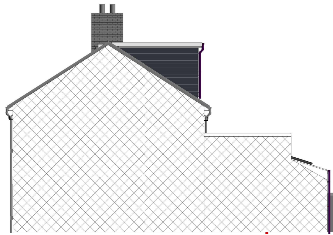
3 SIDE PROPOSED(NW) 1 : 100
