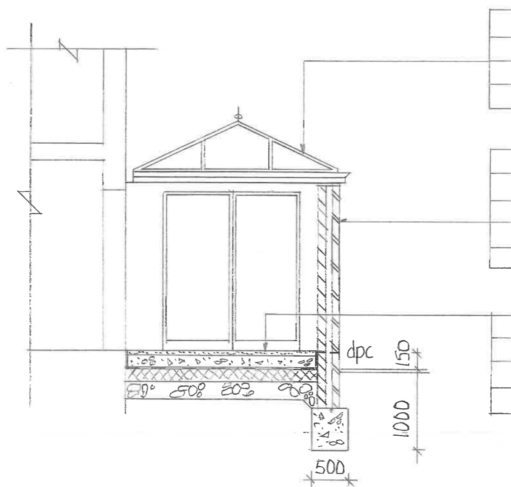
SECTION A-A
