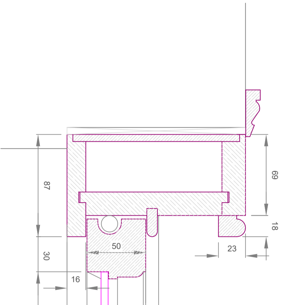
DETAIL A - JAMB SECTION
