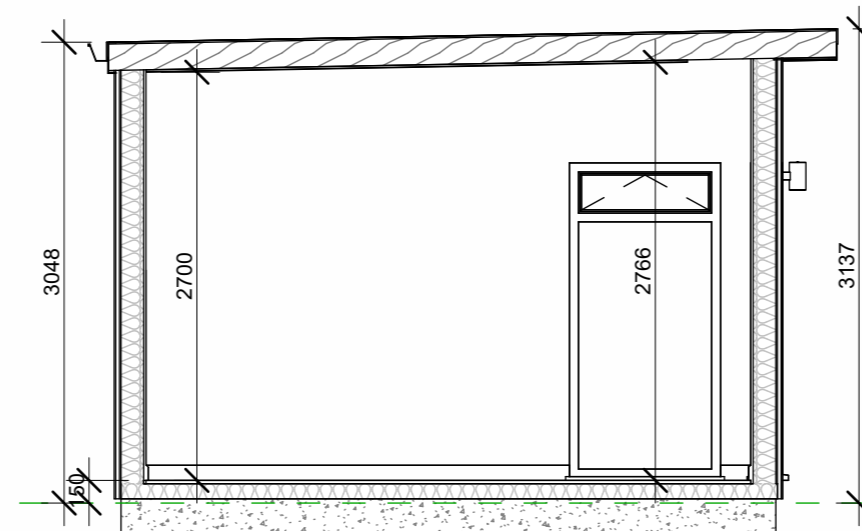
5 Section 1 : 50
