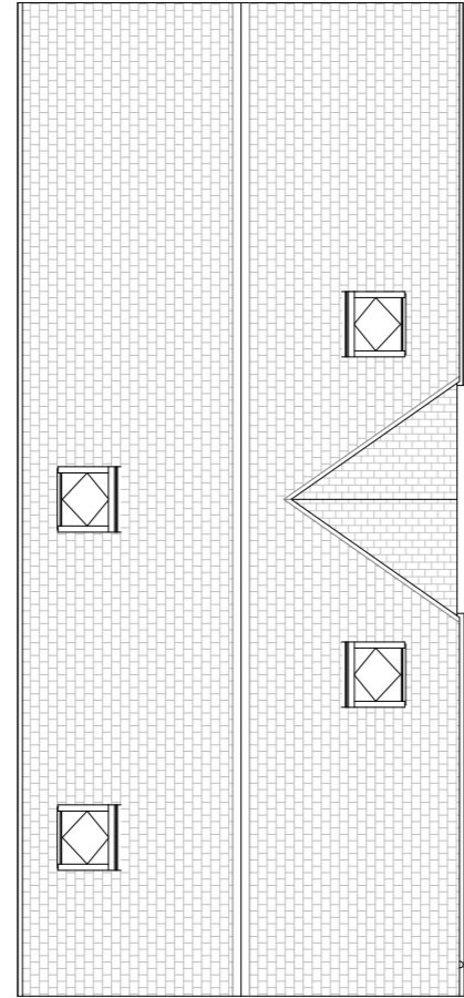
3 Roof Plan 1 : 100
