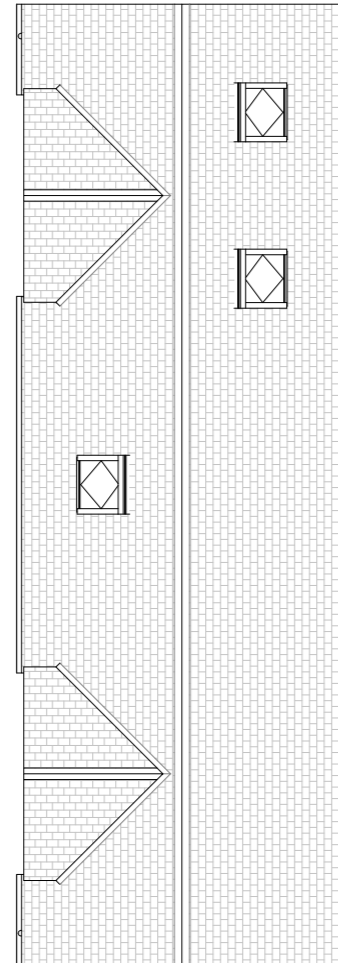
4 Roof Plan 1 : 100
