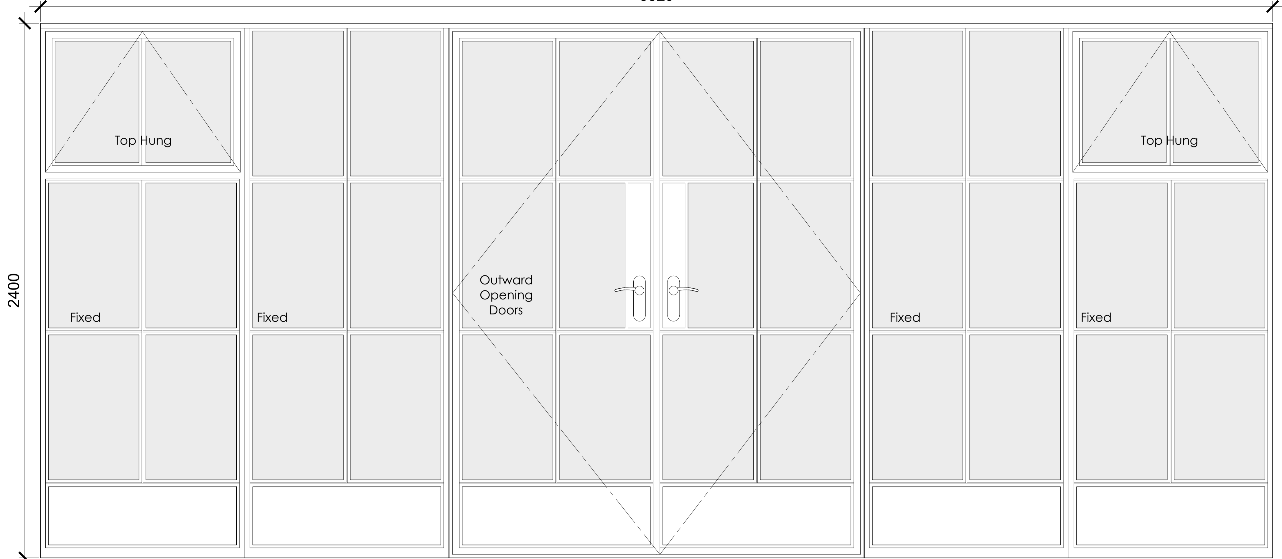
Door Elevation - 1:10
