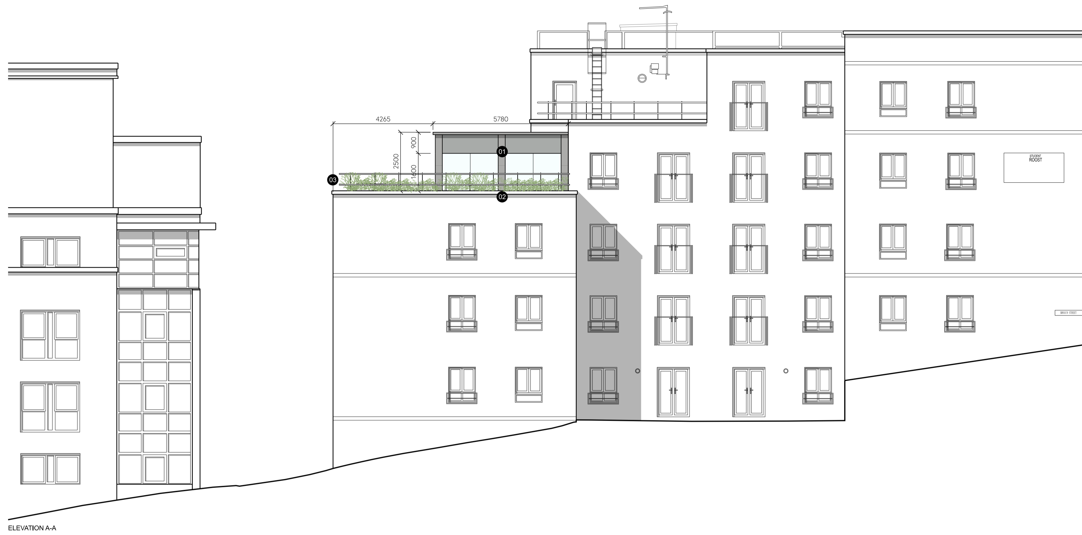
ELEVATION A-A
