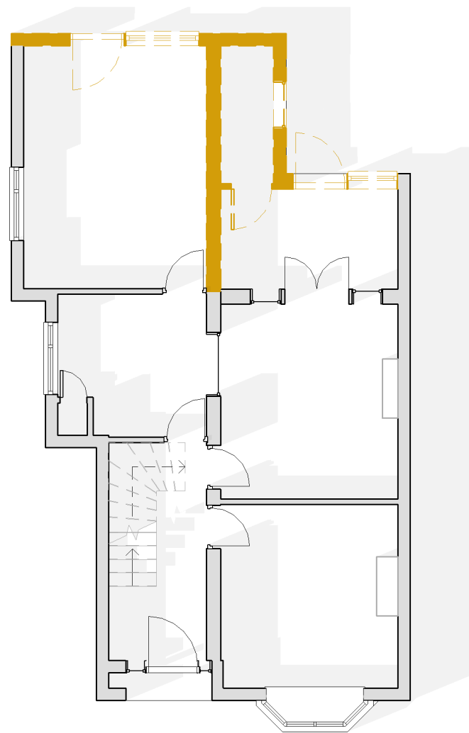
1 0 GF Demo 1 : 100
