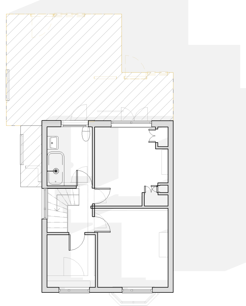
2 1 FF Demo 1 : 100
