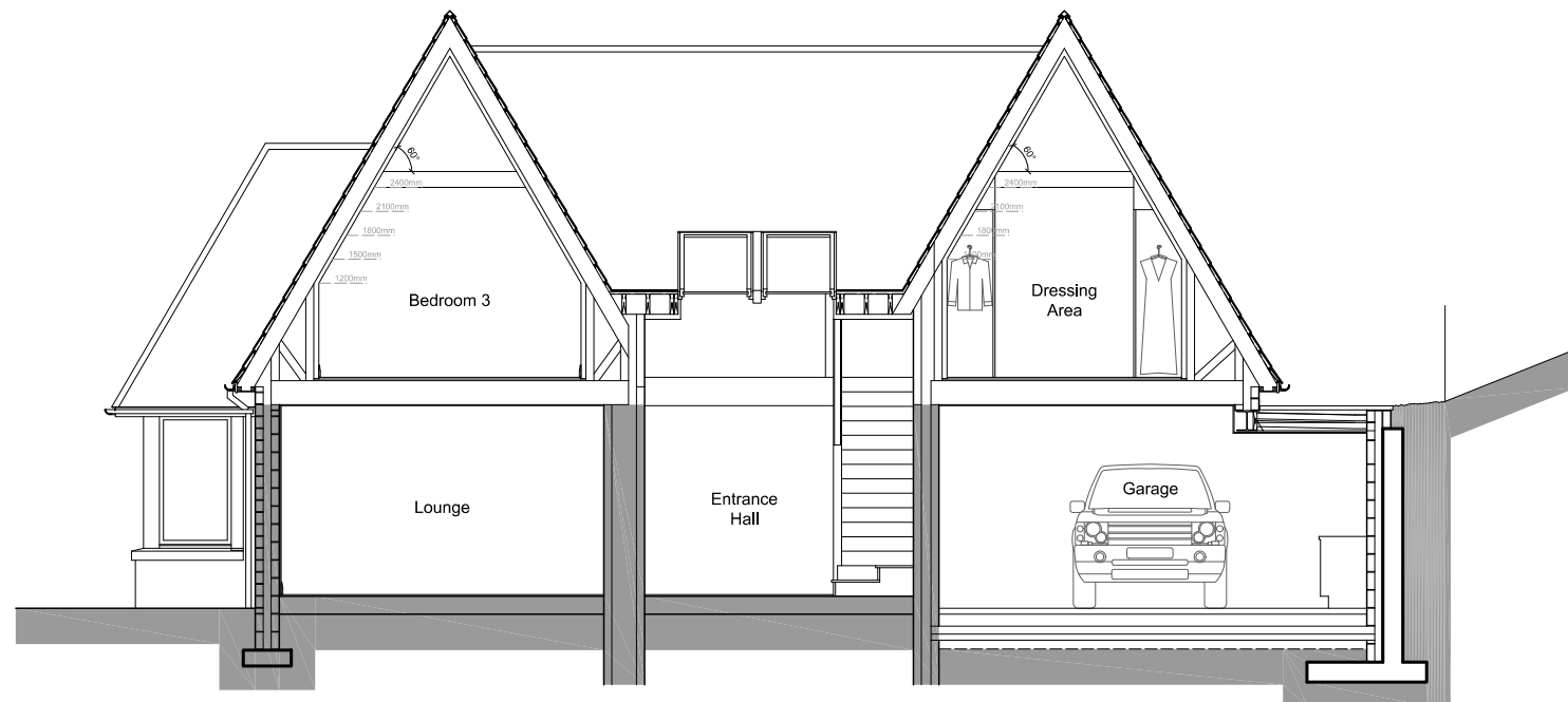
Section A-A
