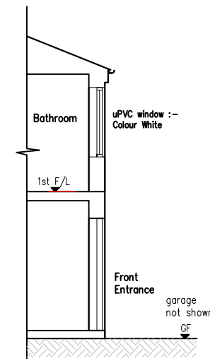
SECTIONAL ELE. 'AA'
