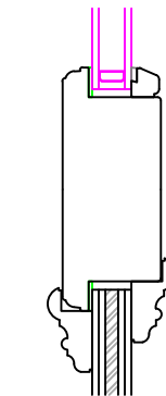
Door Mid Rail
