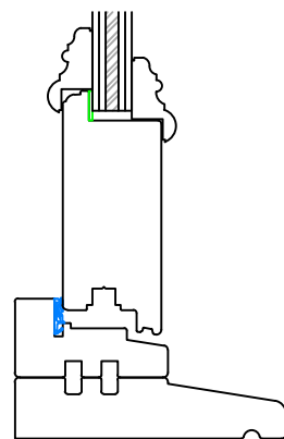
Door Cill
