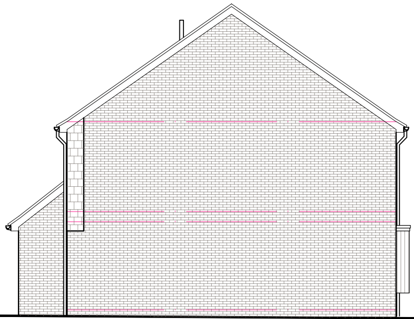
RIGHT FLANK ELEVATION
