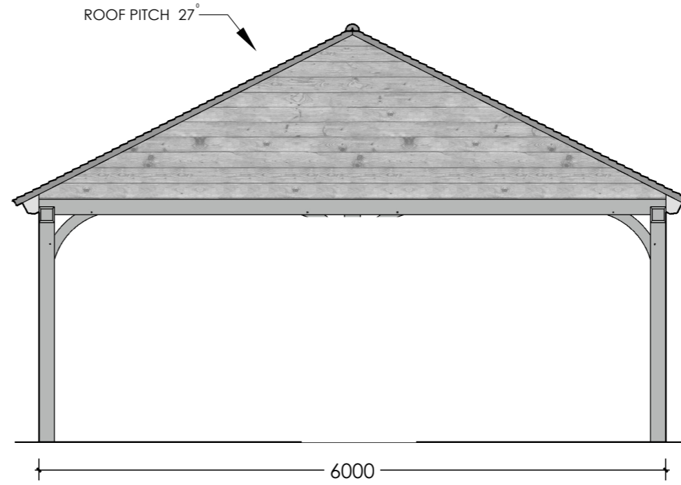
6000 LEFT ELEVATION
