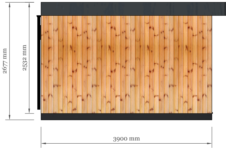
Right Side Elevation - 04 | 1:50 @ A4
