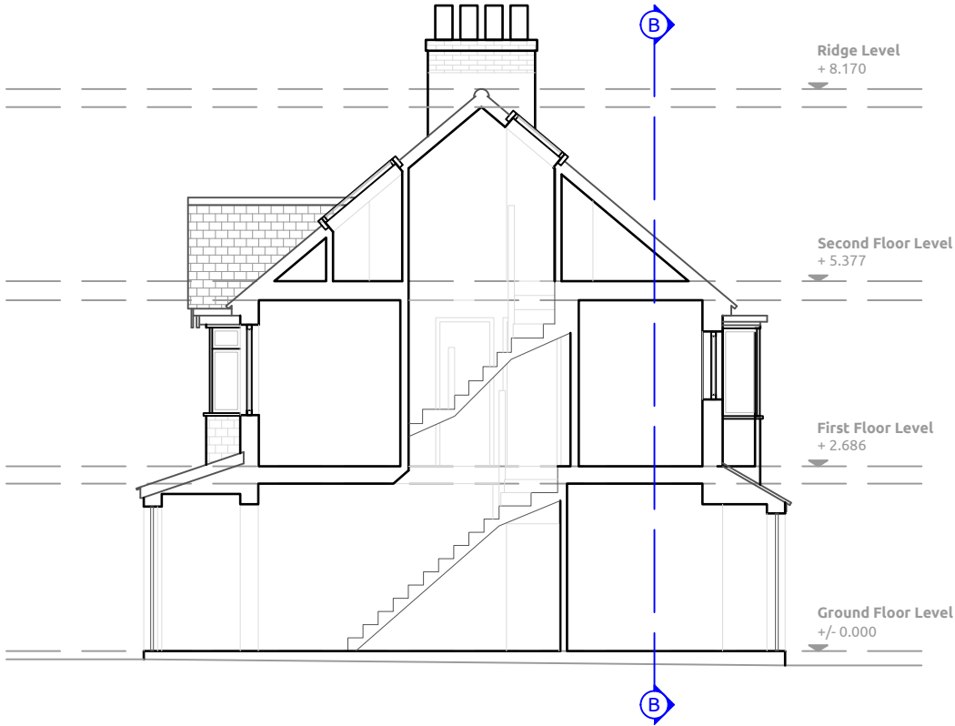
Section A-A
