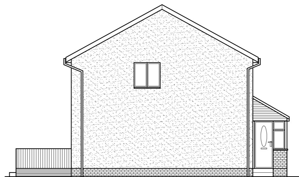
Side 1:100
