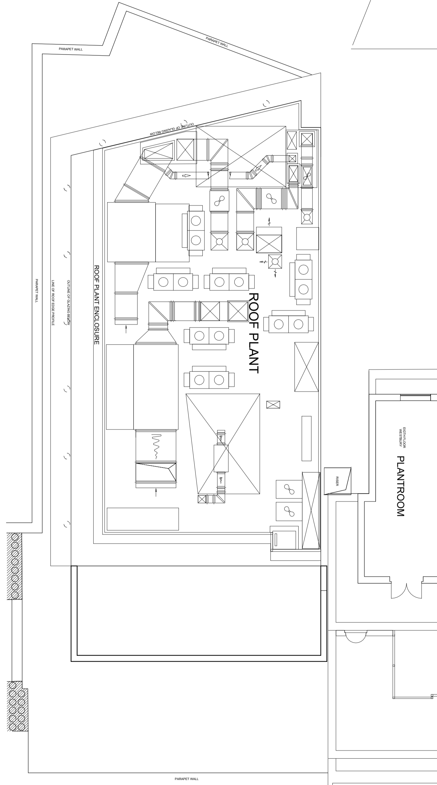
1 07-PLAN Washington. Existing 1 : 100
