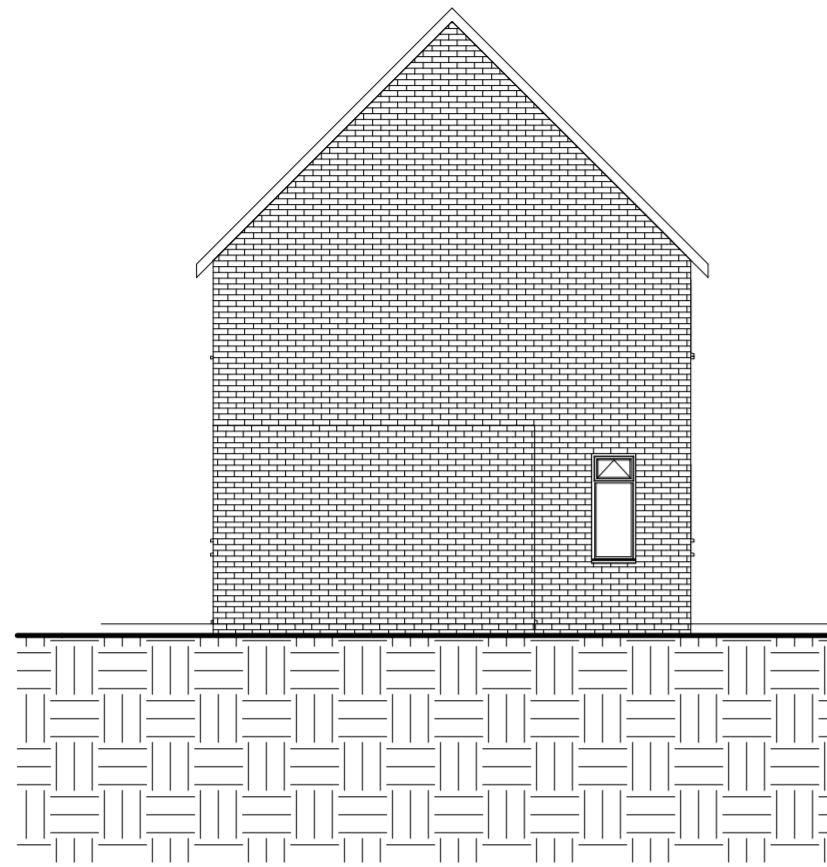
4 North 1 : 100
