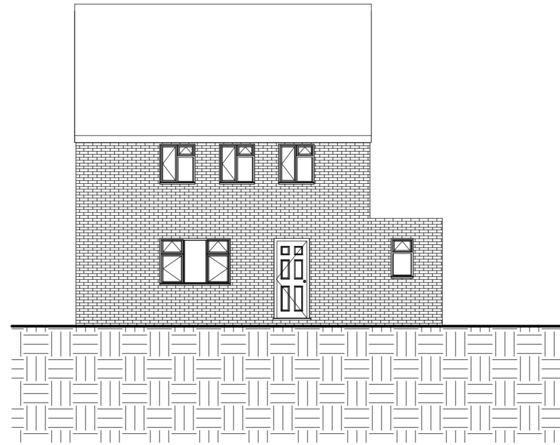
5 East 1 : 100
