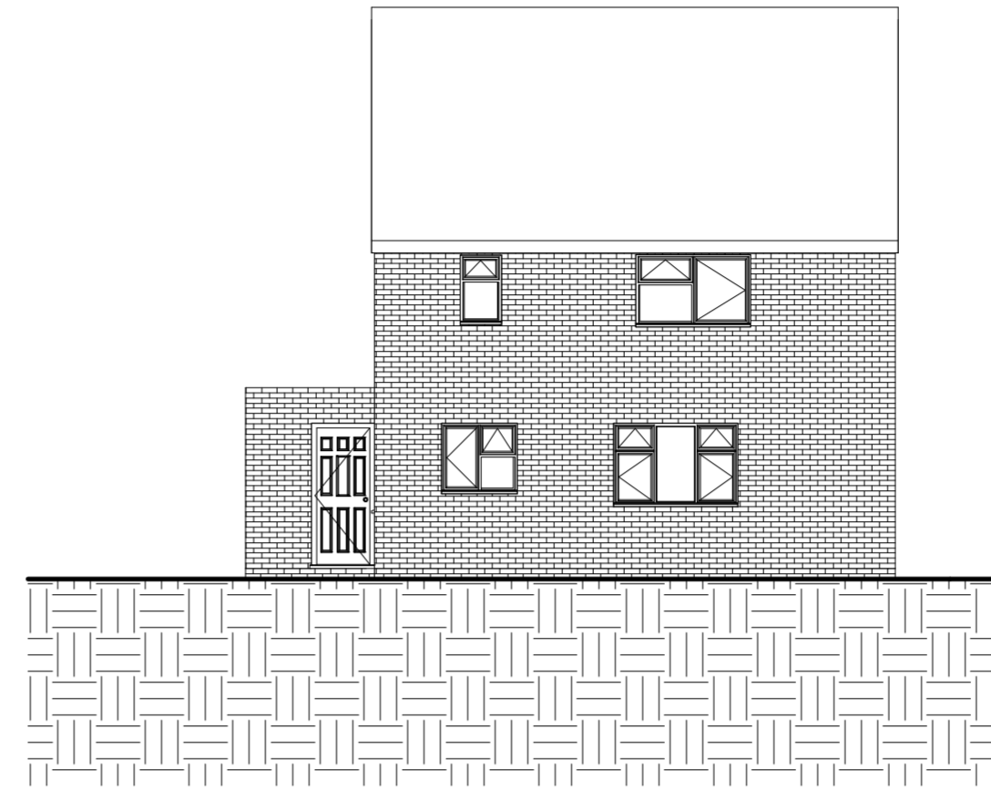
6 West 1 : 100
