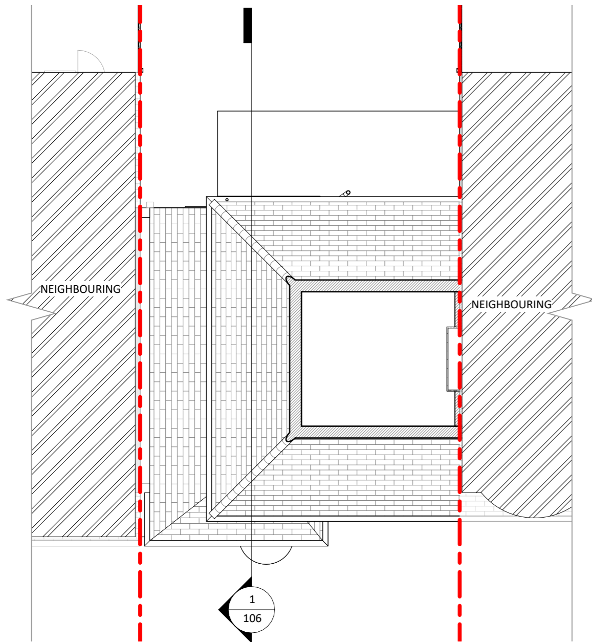
1 Loft (Existing) 1 : 100
