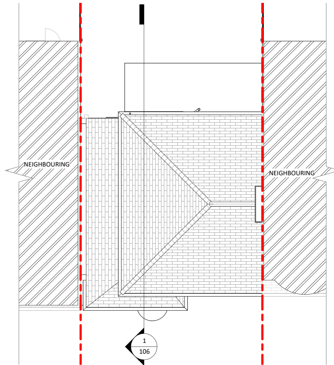
2 Site 1 : 100
