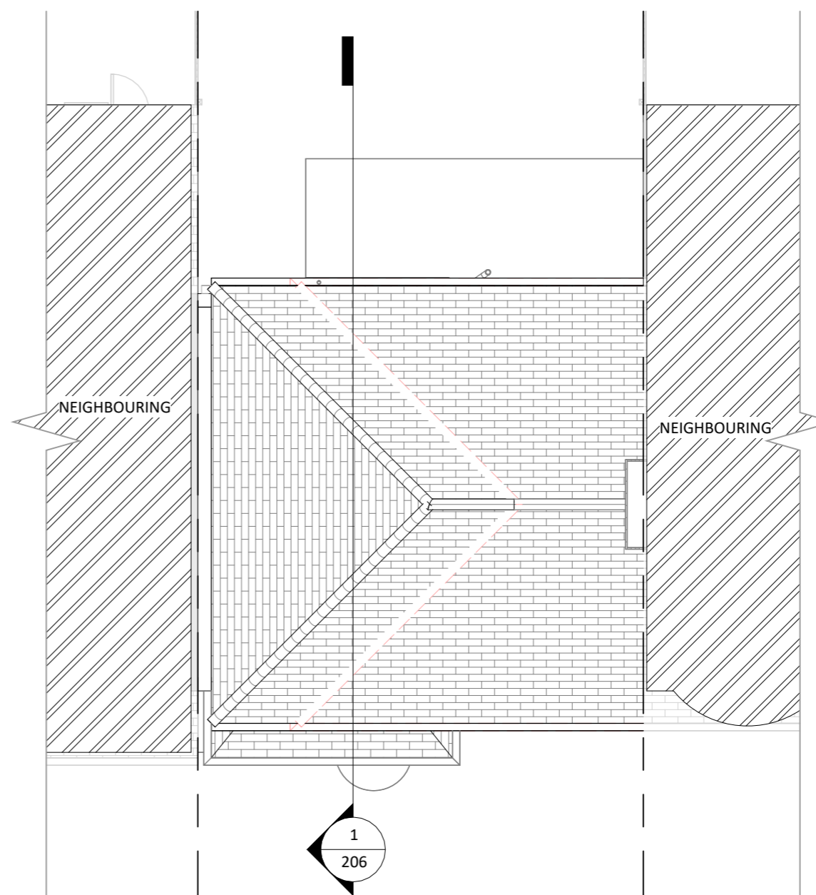
2 Site 1 : 100
