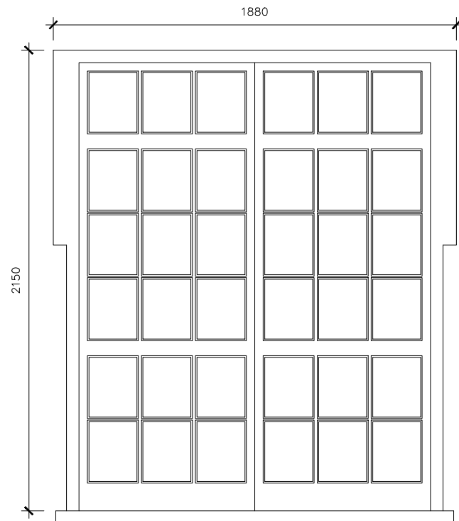
External Door Assembly ED1
