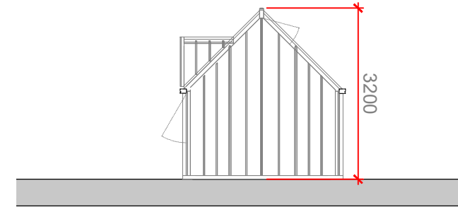
Right Elevation
