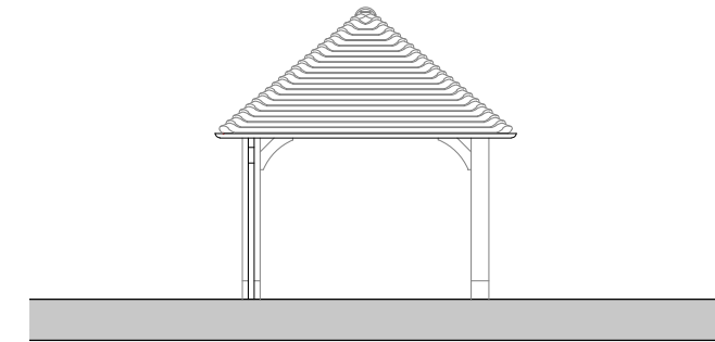
Right Elevation
