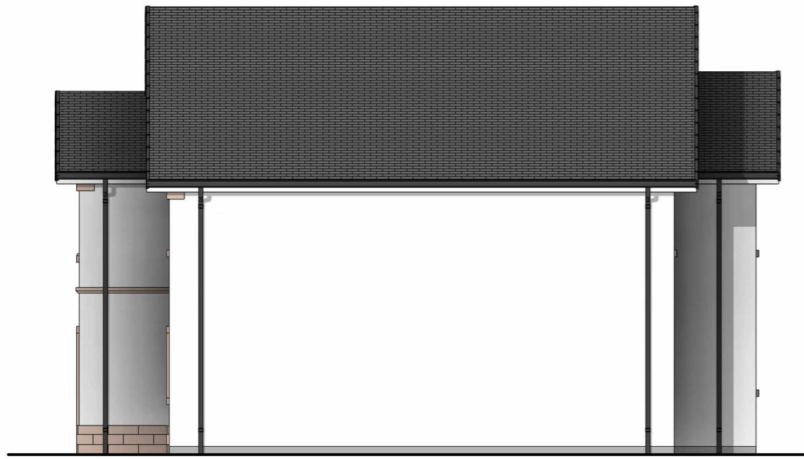
East 1 : 100
