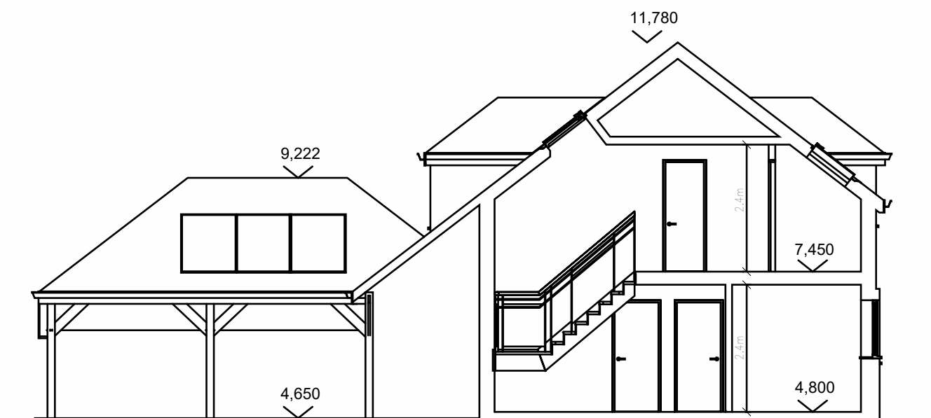
Section 1 : 100
