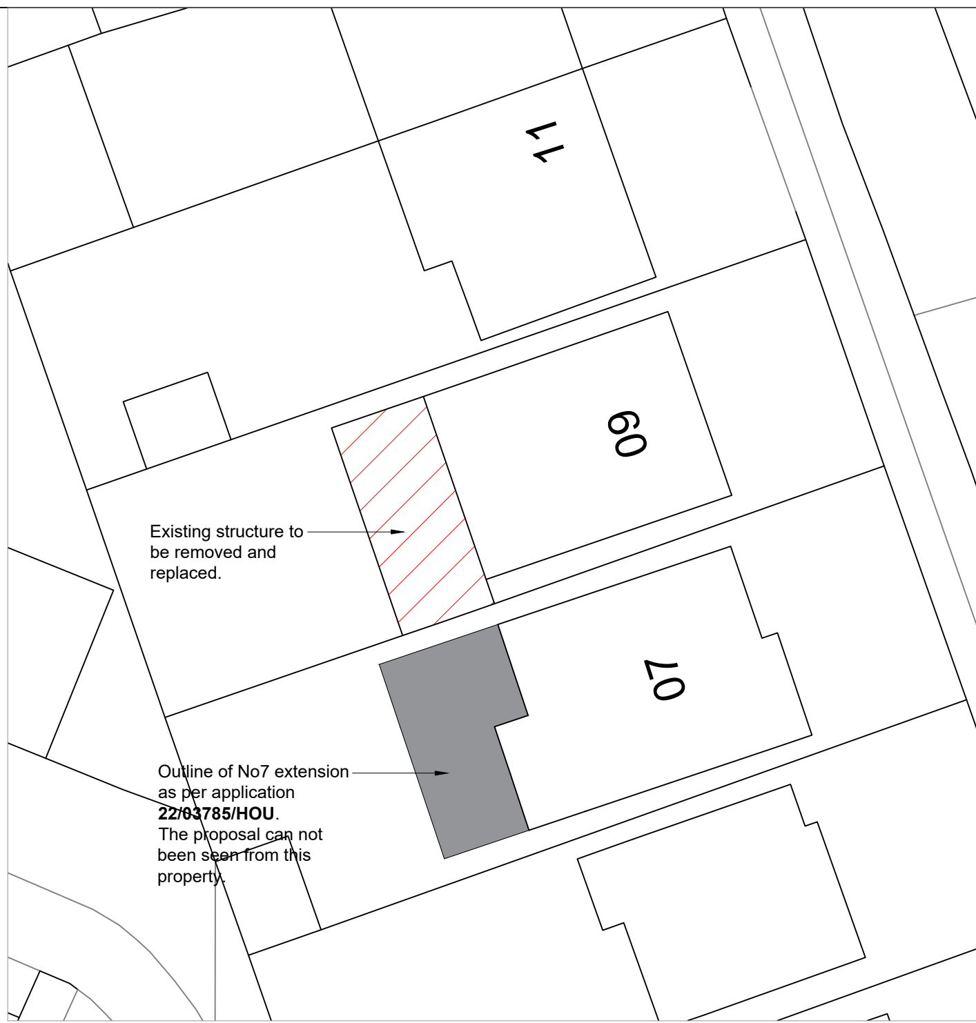
EXISTING SITE PLAN 1:250
