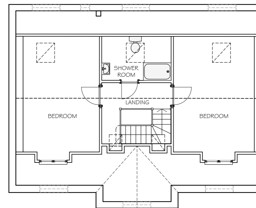
LOFT PLAN
