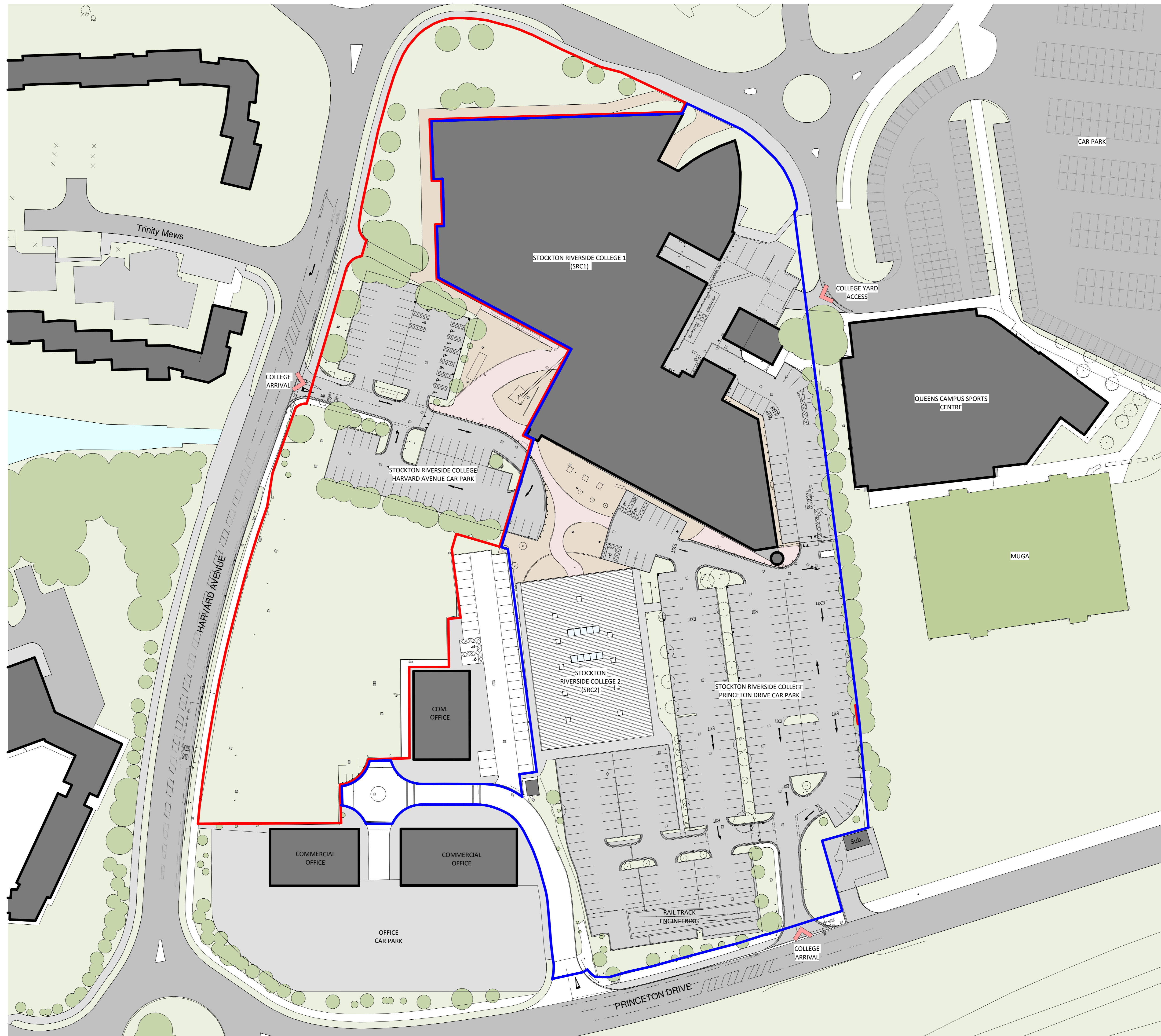
1. Existing Site Plan SCALE - 1 : 500@A3
