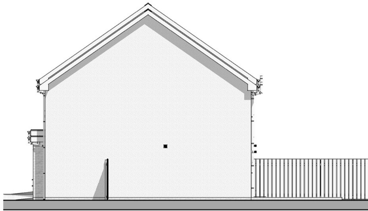
E :: EXISTING SIDE ELEVATION 2 scale: 1:100
