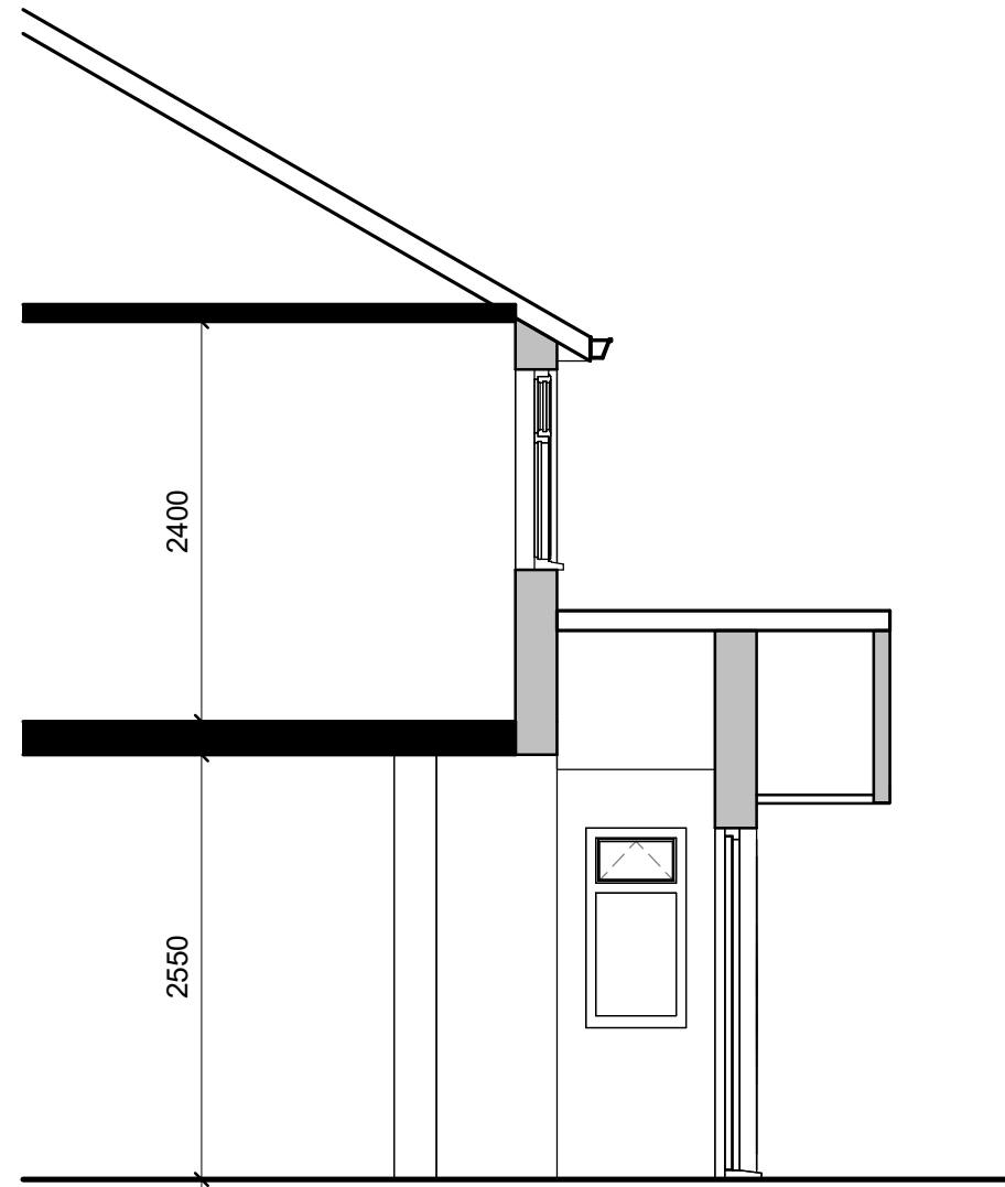
Existing Section 1 1 : 50
