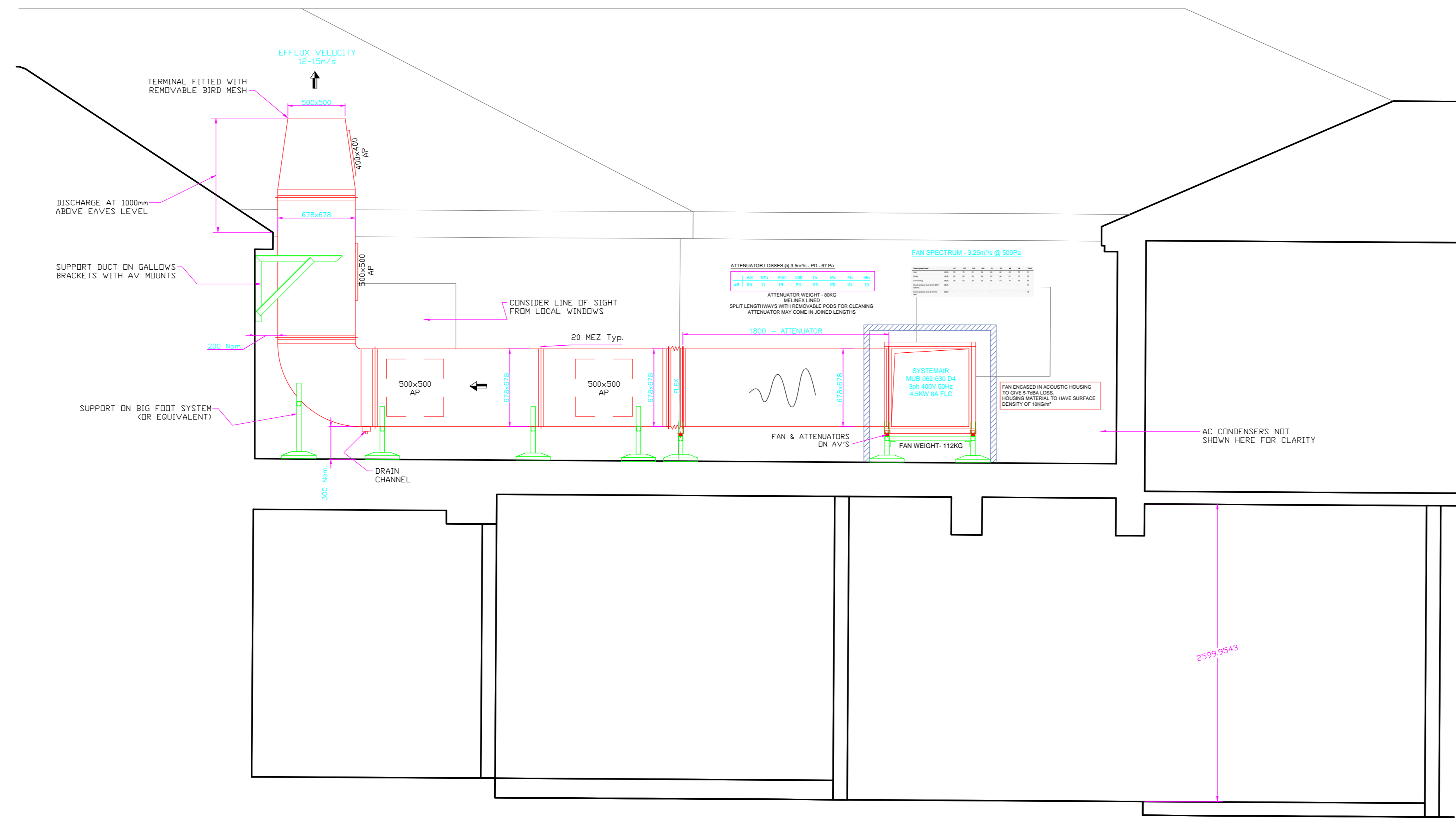
SECTION A-A
