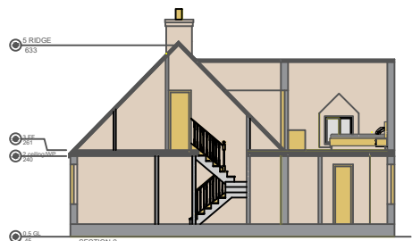
SECTION-2 1:100
